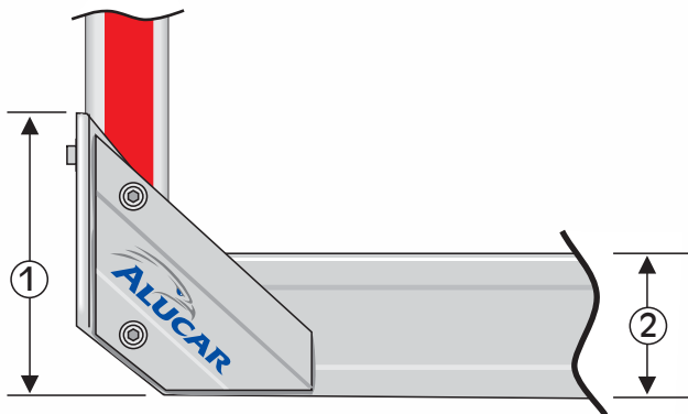
Tolppan kiinnitys pulttaamalla.
