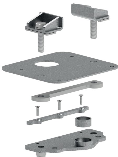
Kiinteä kiinnike
