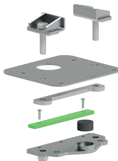
Pikaliukukiinnike
